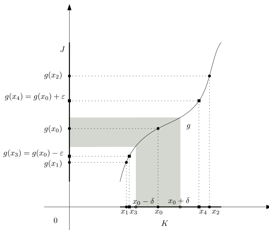
Obrázek 6.1: Pro každé dost malé \varepsilon > 0 najdeme \delta > 0 z vyhovující definici limity. Body x_1 a x_2 omezují, jak velké \varepsilon můžeme uvažovat, abychom zůstali v rámci intervalů J a K . Toto omezení na \varepsilon nám ale nevadí, protože pokud najdeme \delta pro malé \varepsilon , tato hodnota \delta funguje i pro všechna větší \varepsilon .
