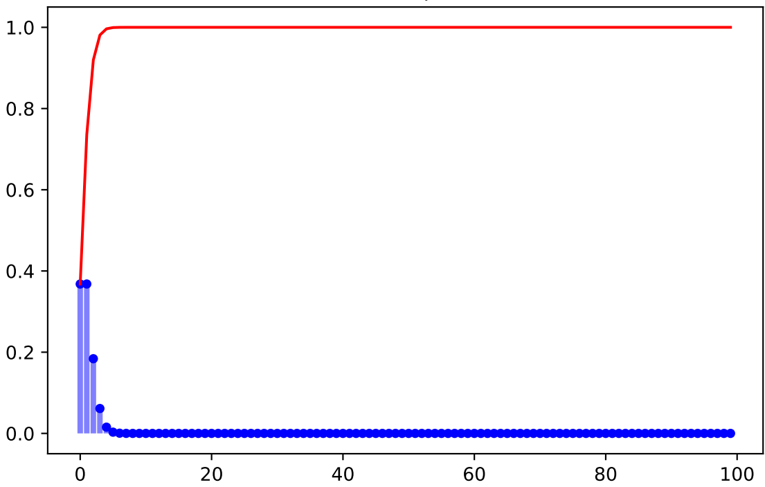
Poisson( \mu=5 )
