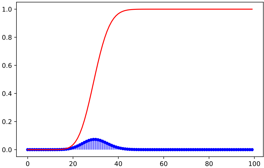
Poisson( \mu=30 )
