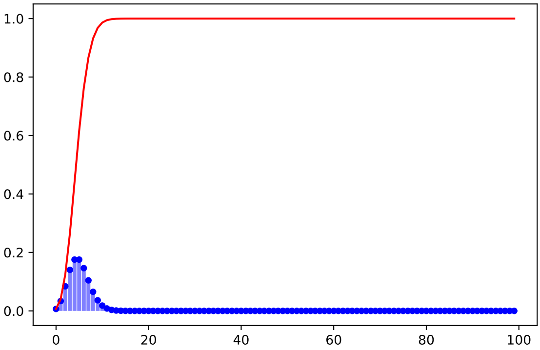
Poisson( \mu=5.0 )
