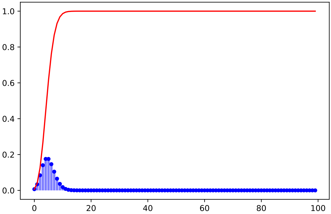
Poisson( \mu=5.0 )
